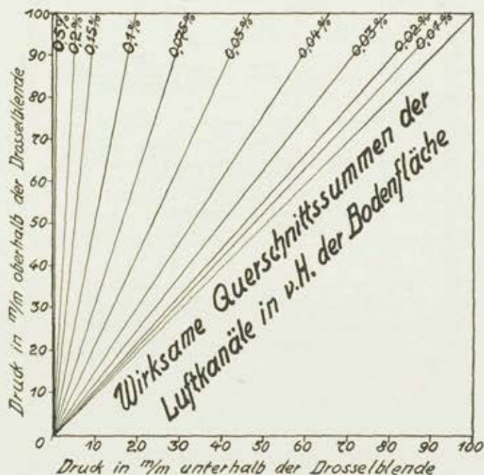
Abb. 2. Eichtafel zur graphischen Ermittlung der Durchlüftbarkeit des Bodens
