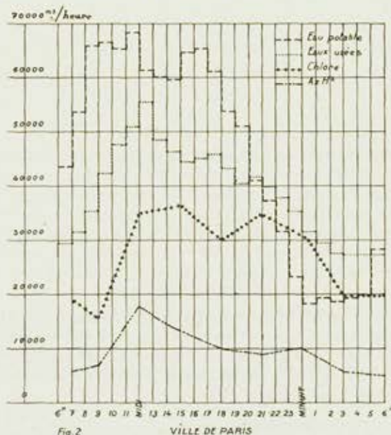
Variation des débits en eau potable et en eau usée et de la composition de celle-ci dans le cours d'une même journée (D'après Sentenac)
