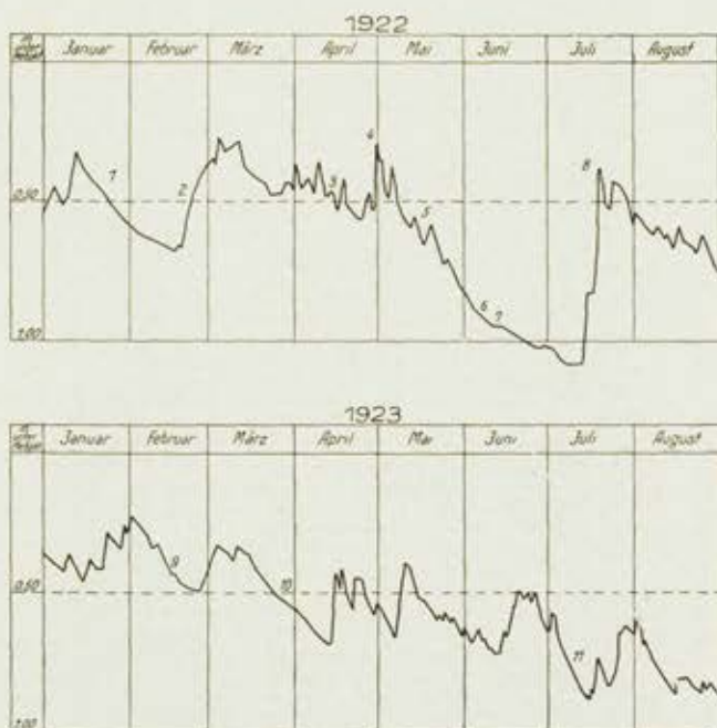
Abb. 1: Grundwasserstände in einem Niederungsmoor in Berlin-Zehlendorf.
