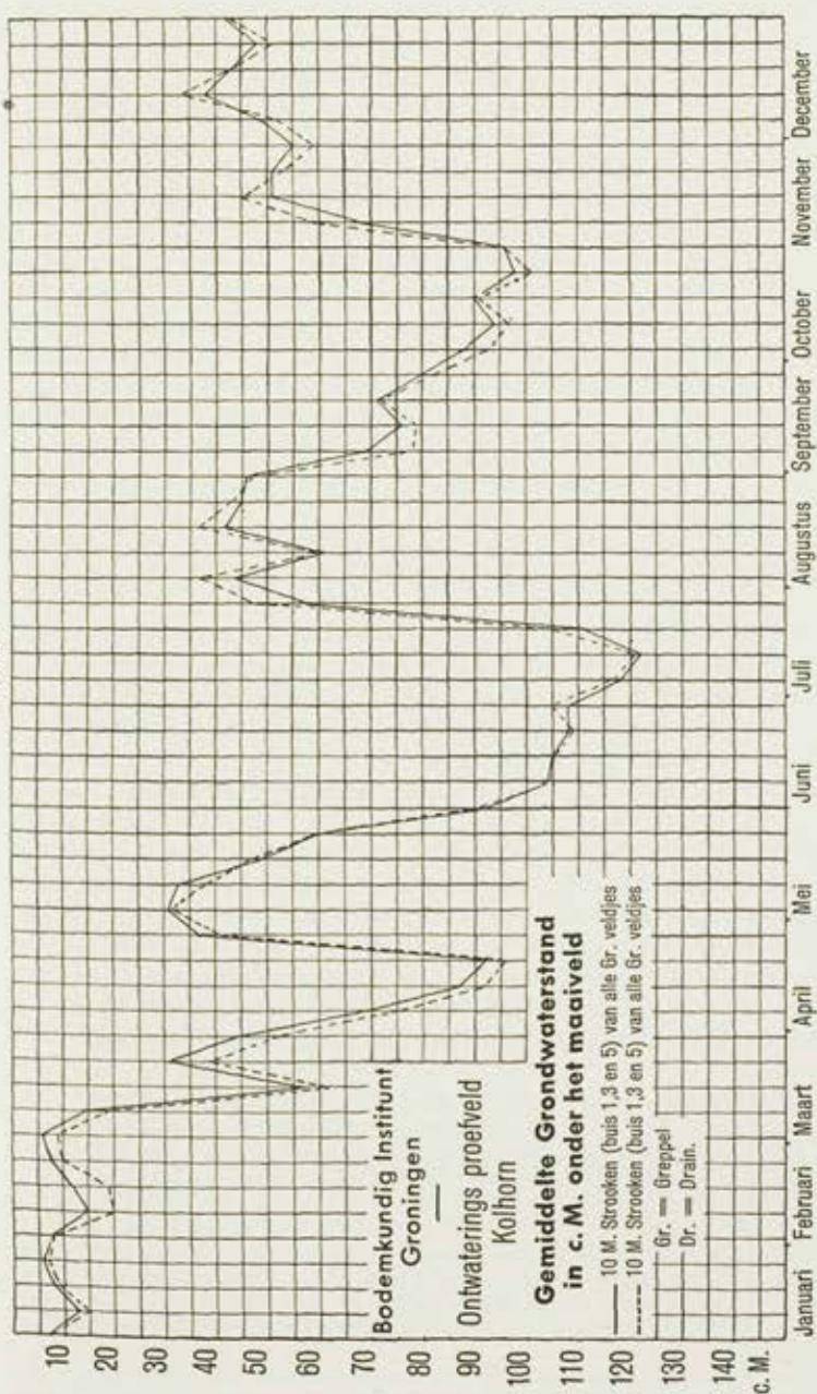
Abb. 2. Erläuterung: Alle Grundwasserstände sind in cm unter der Erdoberfläche (Nied.: Maaveld) angegeben. — Grundwasserstand in der Mitte zwischen offenen Gräben mit einer Grabenentfernung von 10 m. - - - Grundwasserstand in der Mitte zwischen Dränsträngen mit einer Strangentfernung von 10 m.
