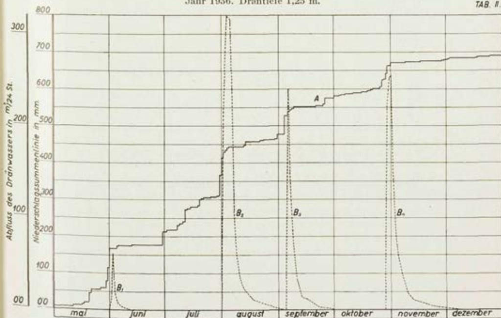
NIEDERSCHLAGSSUMMENLINIE, A 1 UND DIE ABFLUSSMENGEN DES DRÄNWASSERS, B 1 , B 2 , B 3
